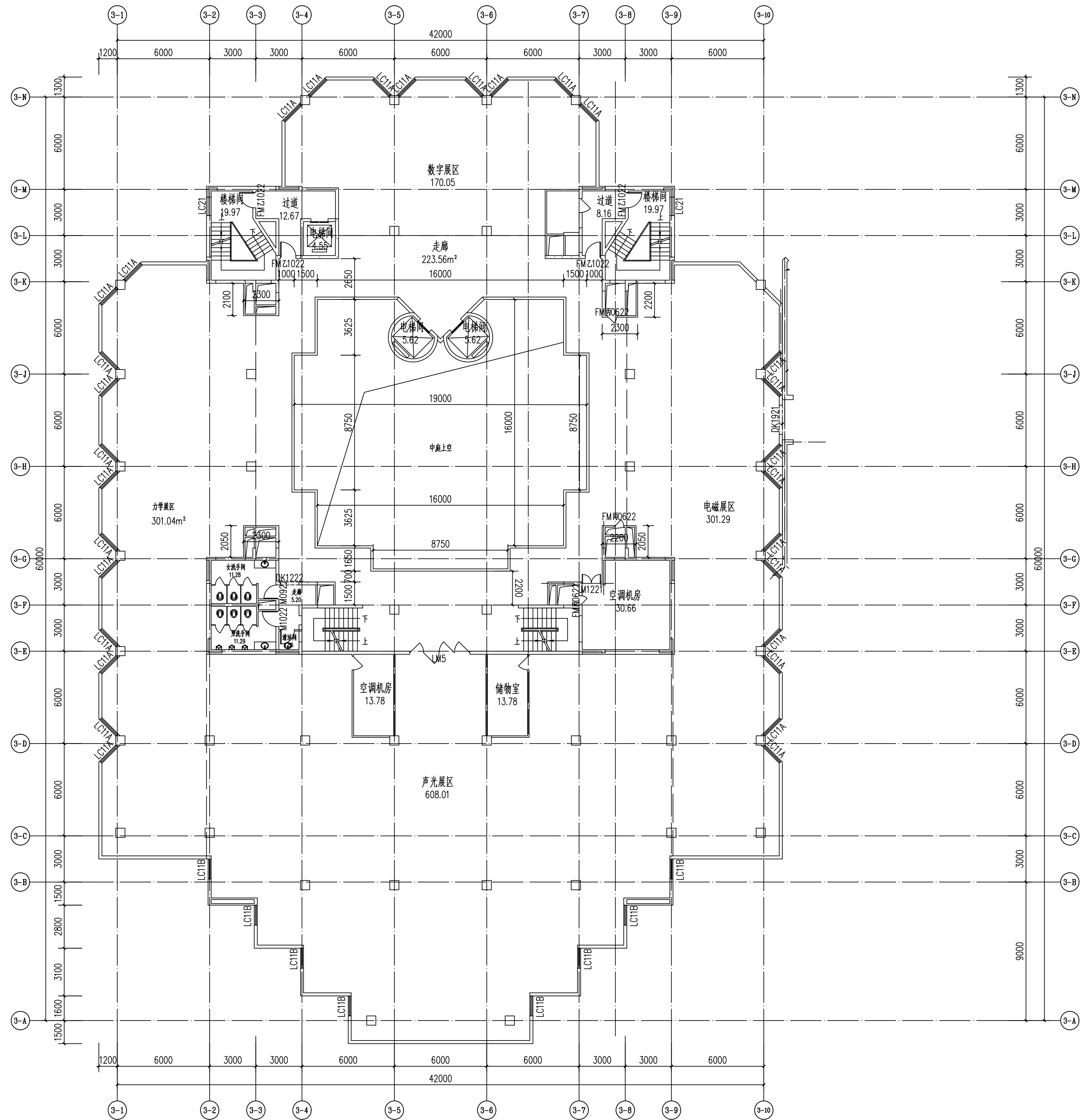
二层平面图 1:150
